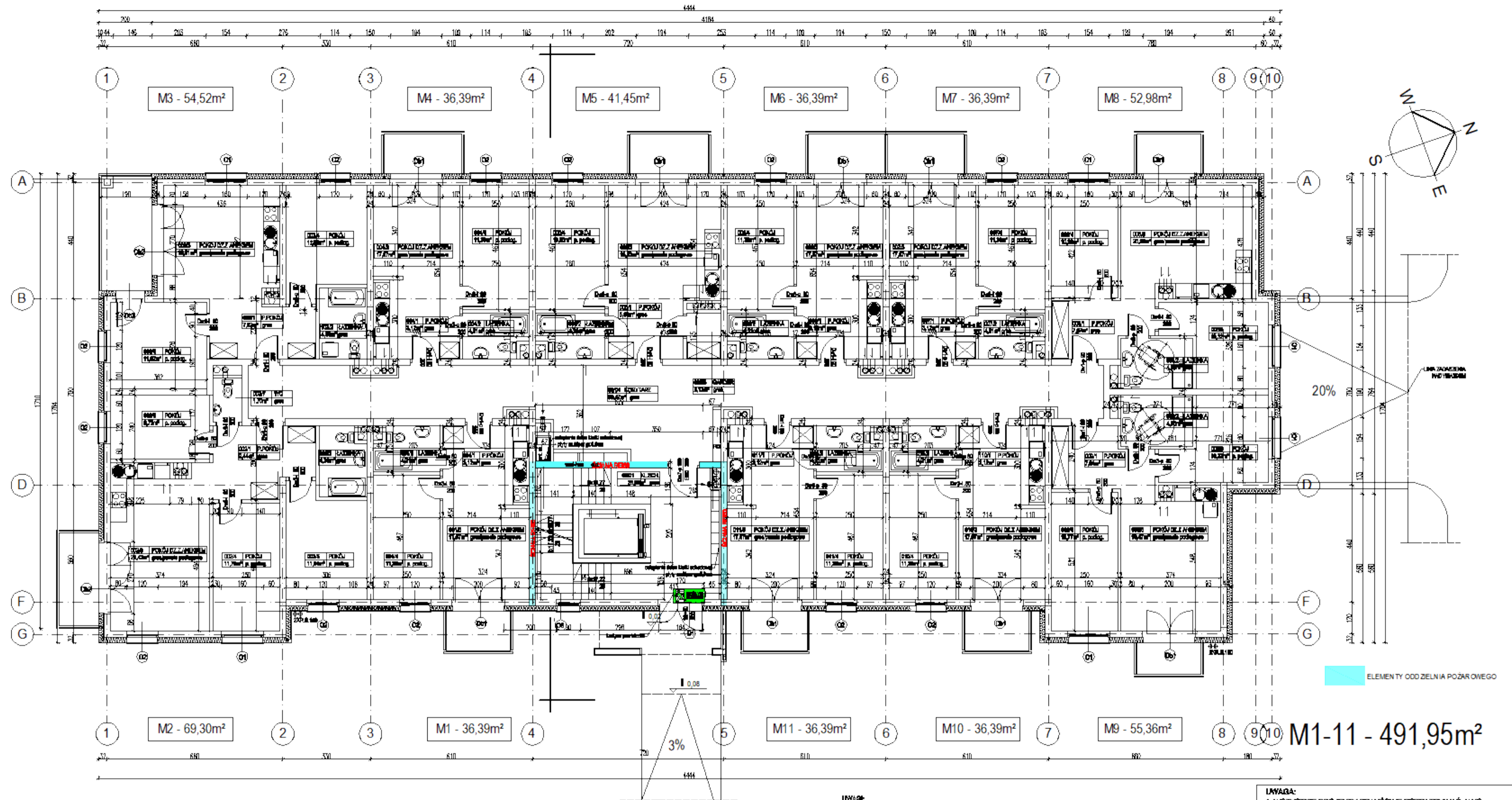
RZUT PARTERU 1:100
