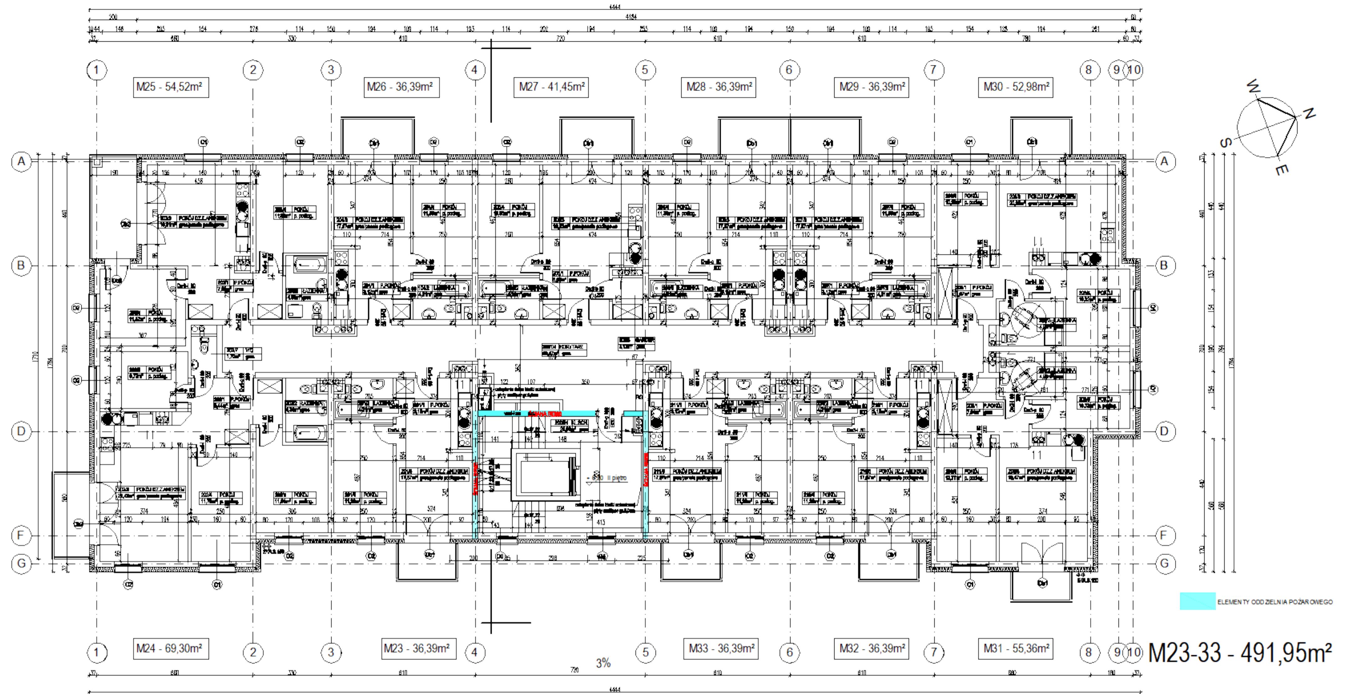
RZUT II PIĘTRA 1:100
