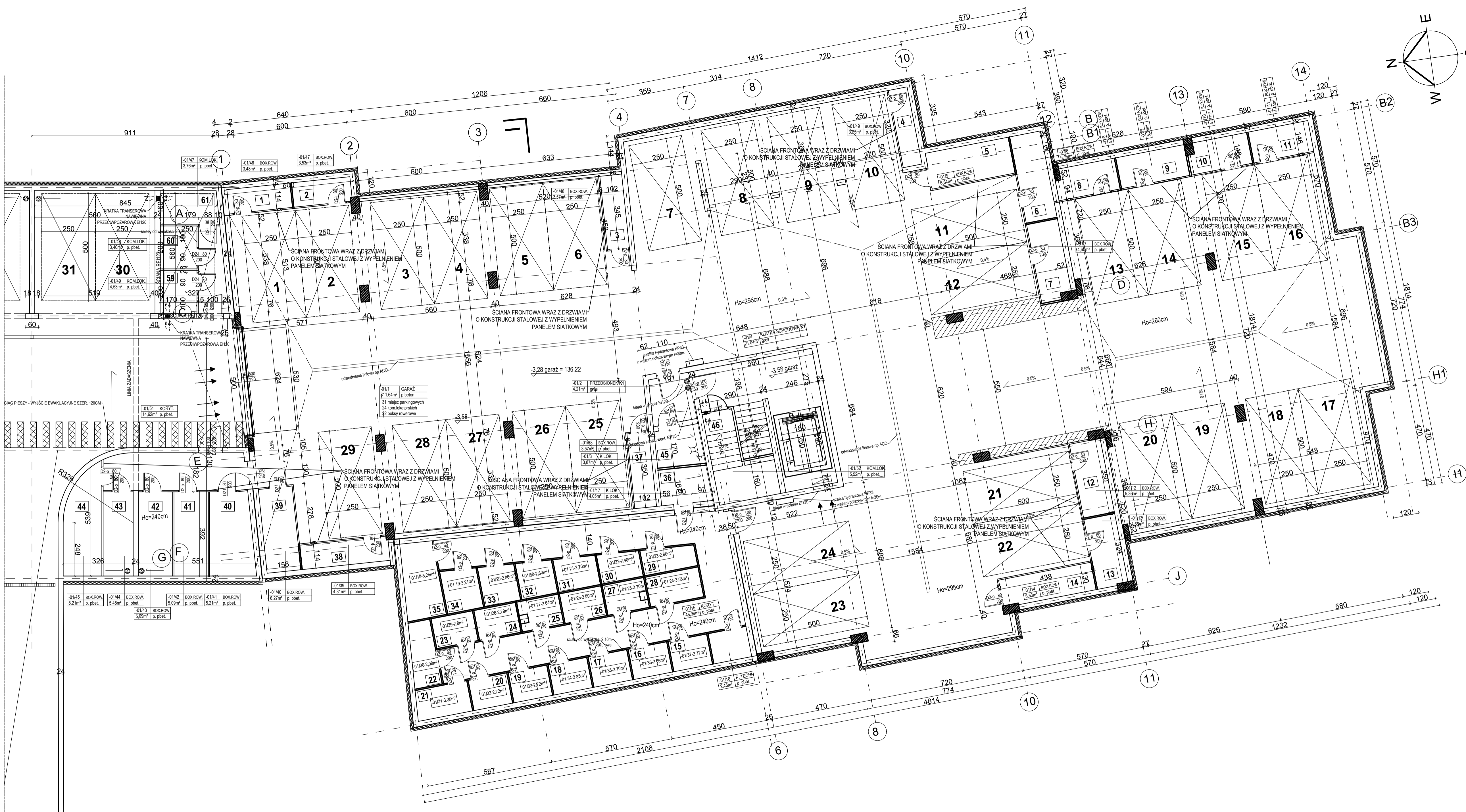
RZUT GARAŻU 1:100 BUDYNEK NR 24
